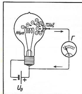
Σχ. 438. "Όταν ή πλάξ συνδέεται, μέσω του ελασθήτου γαλβανόμετρου, προς τόν θετικόν πόλον πηγής συνεχούς τάσεως, τὰ ήλεκτρόνια κινούνται εκ τού διαφόρου νήματος προς τήν πλάκα."
